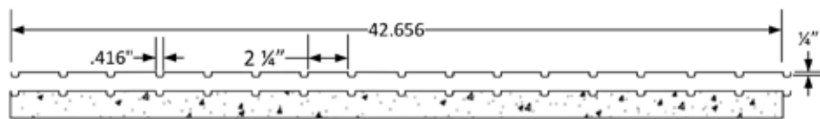
Section A-A
