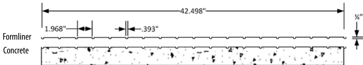
Section A-A
