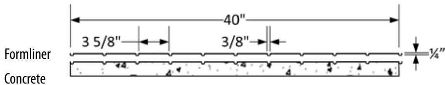
Section A-A
