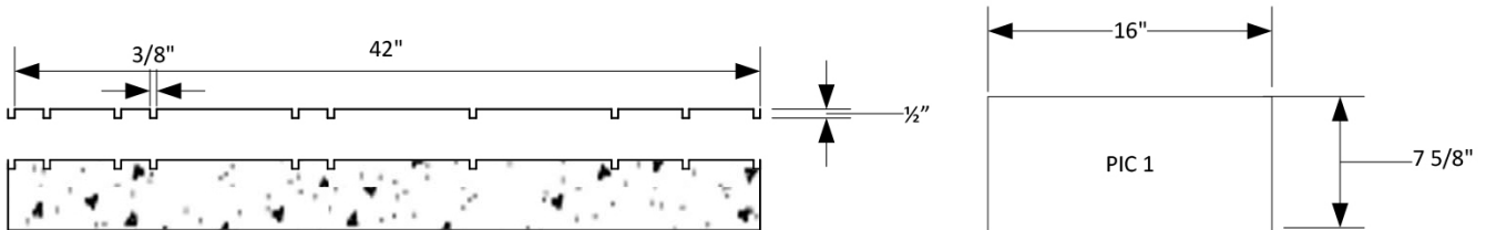
Section A-A
